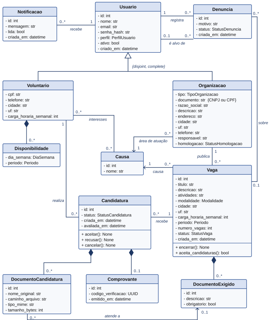
Figura 7 – Diagrama de classes do domínio
