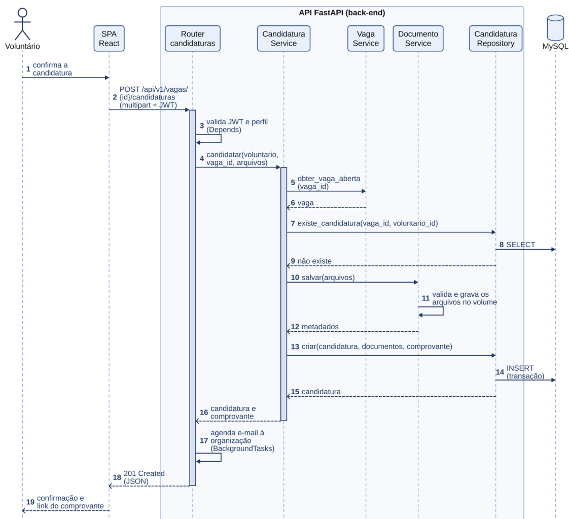
Figura 2 – Interação entre as camadas na candidatura a uma vaga (diagrama de sequência)
