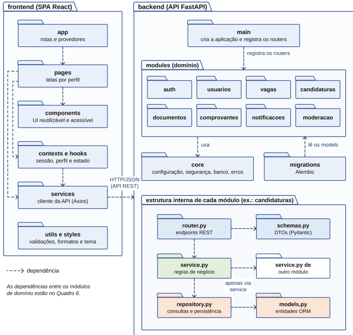
Figura 5 – Diagrama de pacotes do VolunJá
