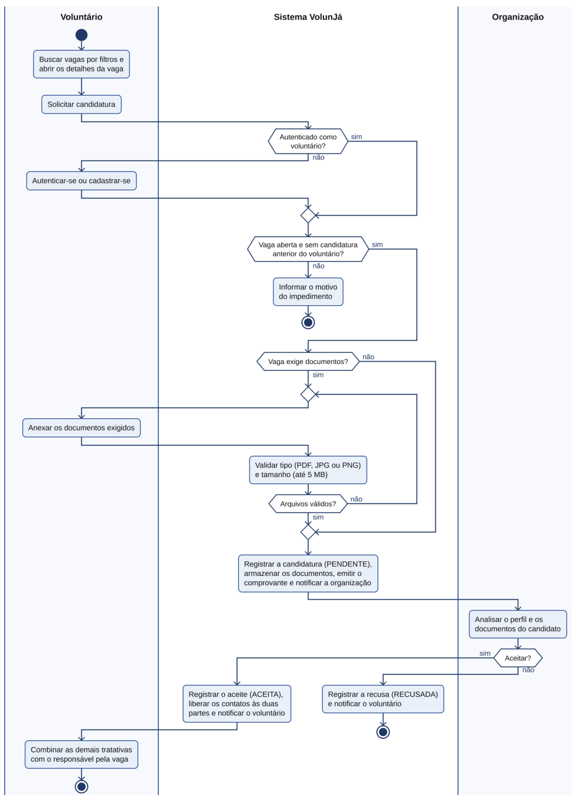
Figura 4 – Diagrama de atividades da candidatura a uma vaga
