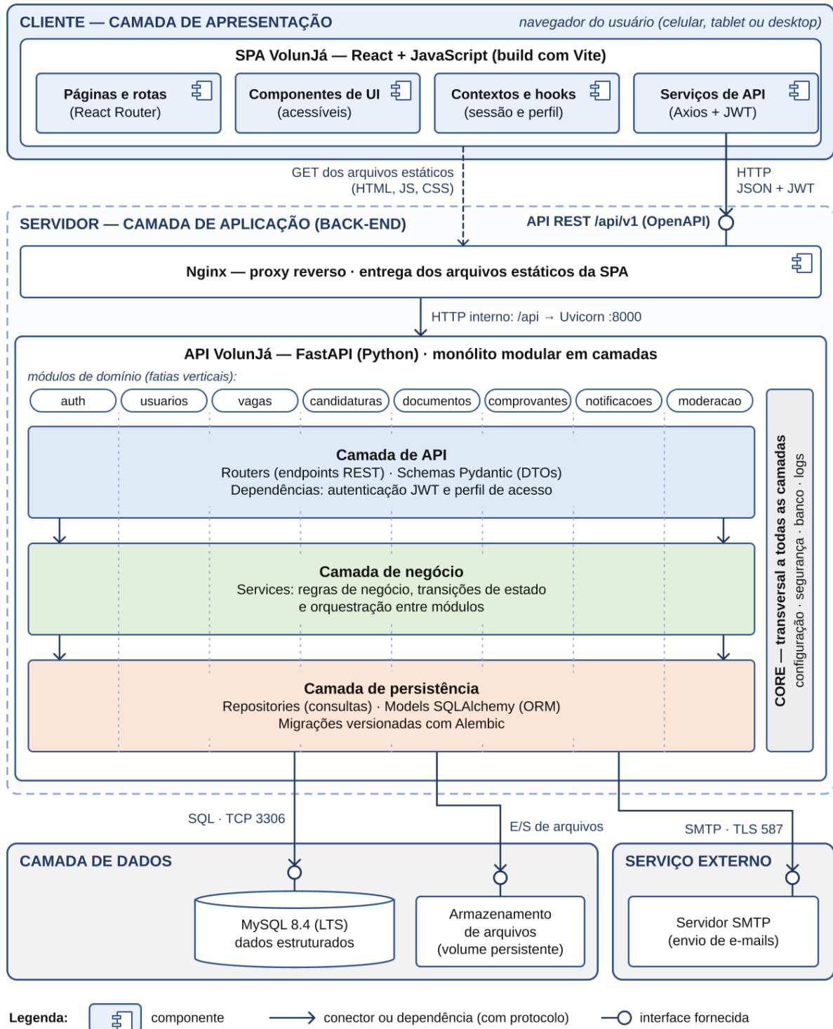
Figura 1 – Representação esquemática da arquitetura do VolunJá
