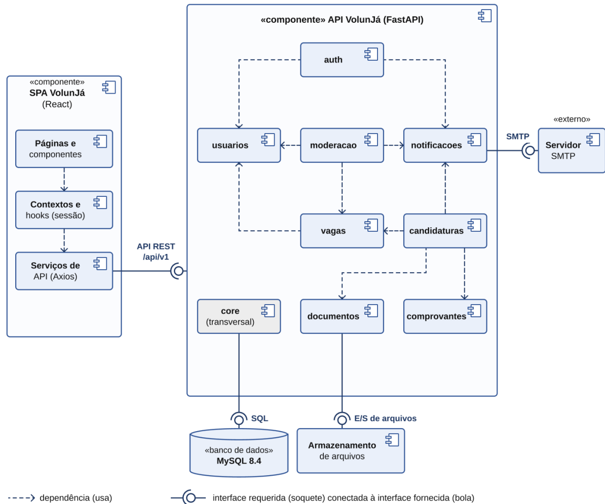
Figura 6 – Diagrama de componentes do VolunJá
