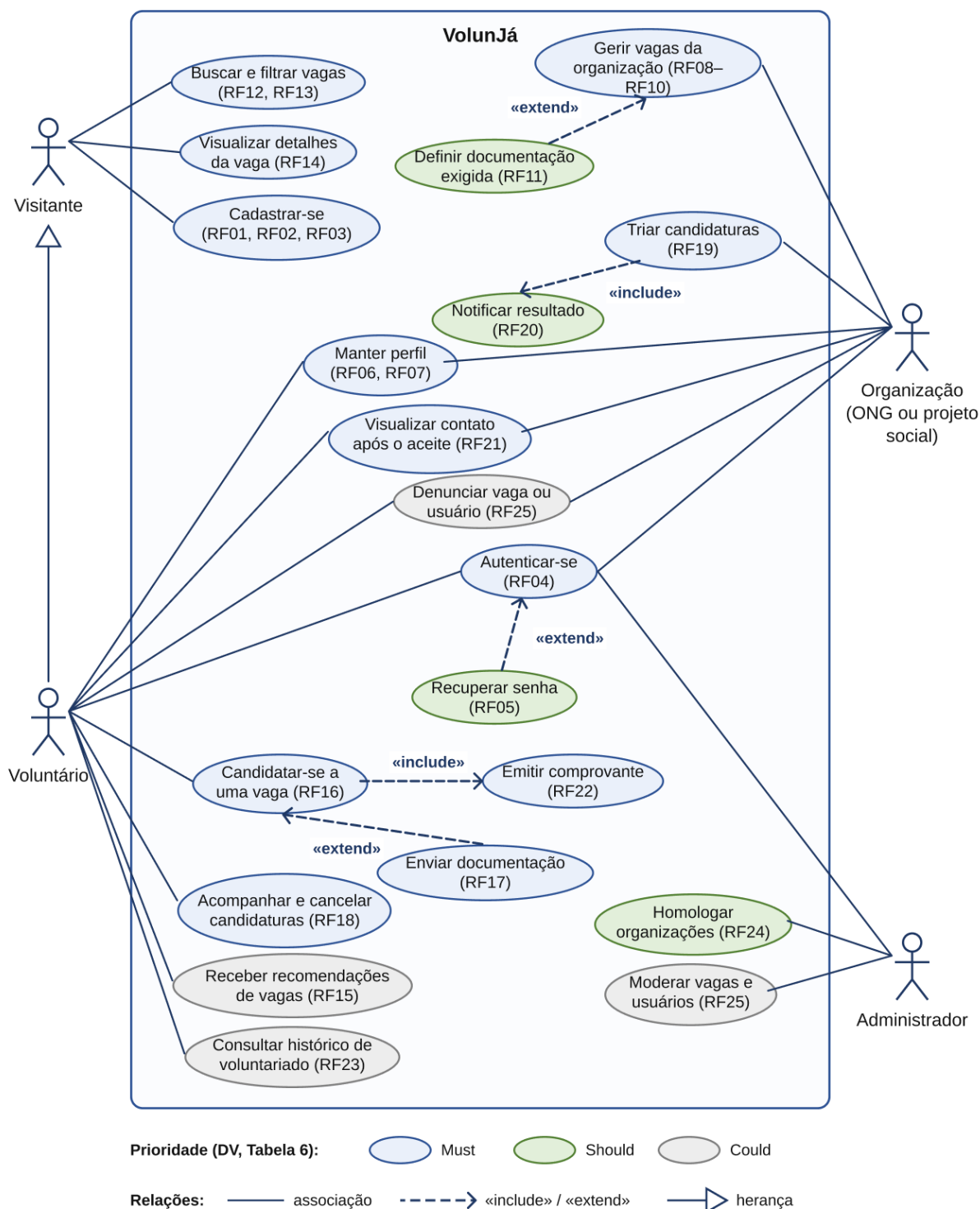
Figura 3 – Diagrama de casos de uso do VolunJá
