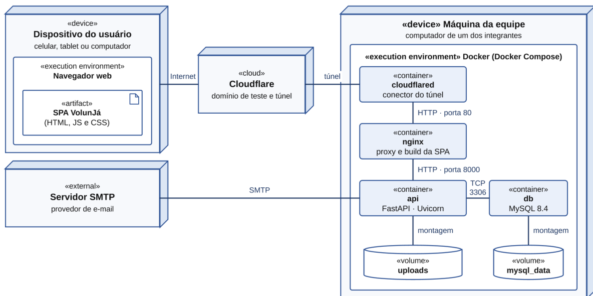
Figura 8 – Diagrama de implantação do VolunJá
